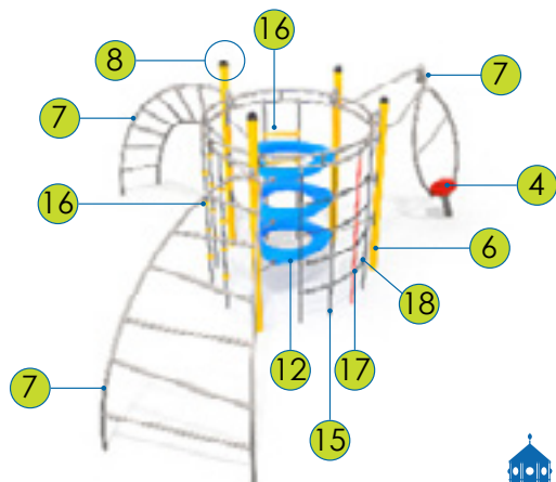
16 Taustige og tauknuter av støpt polyamide.
